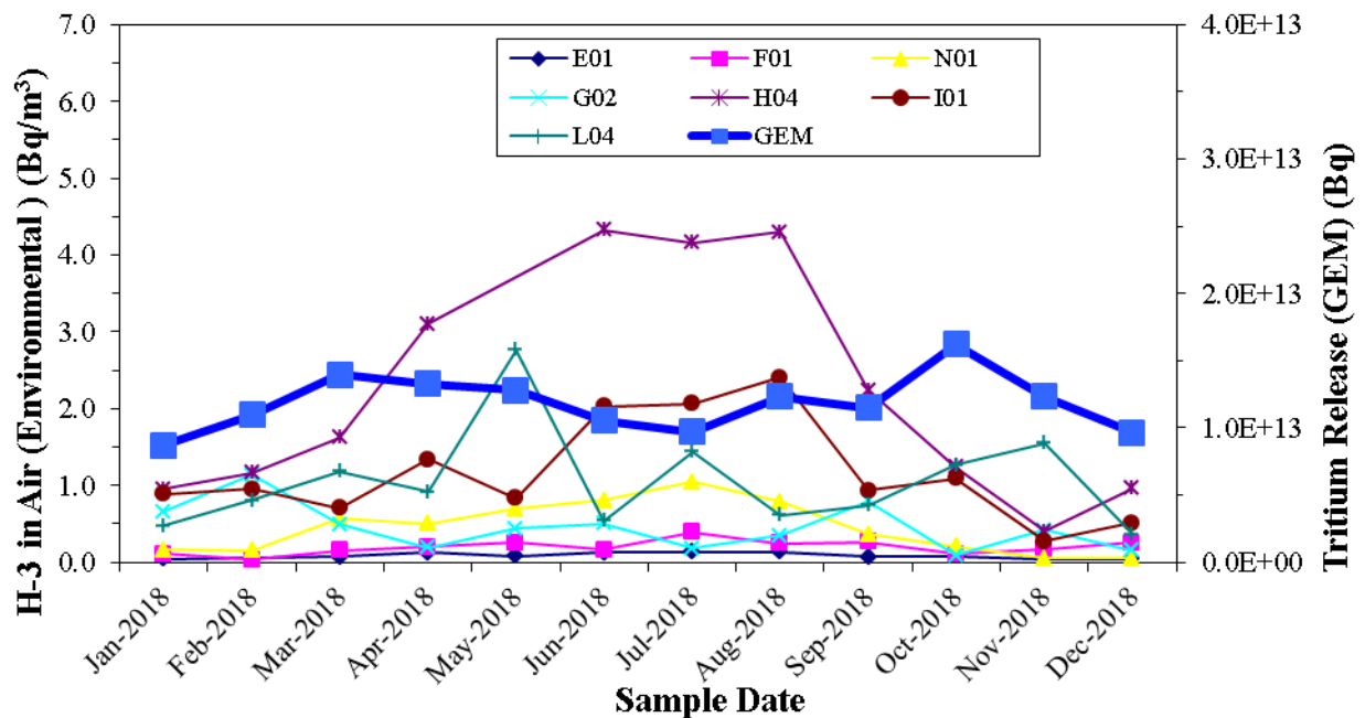
Image 4.06: Résultats relatifs aux émissions de H-3 gazeux et de H-3 (vapeur d'eau)
