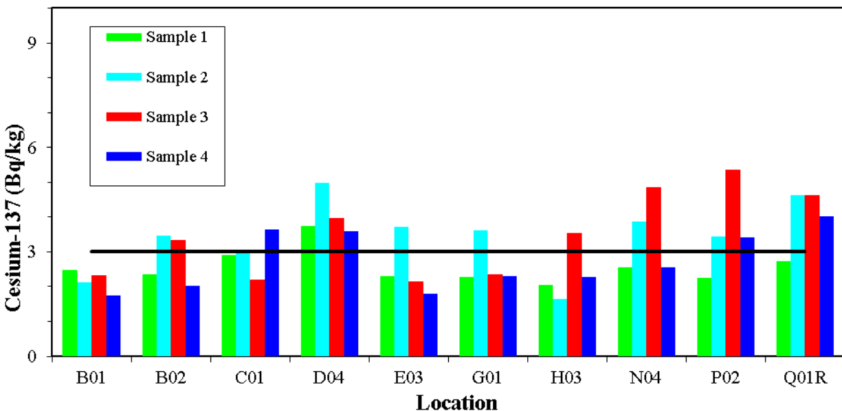
Image 4.19: Césium-137 (sédiments)
