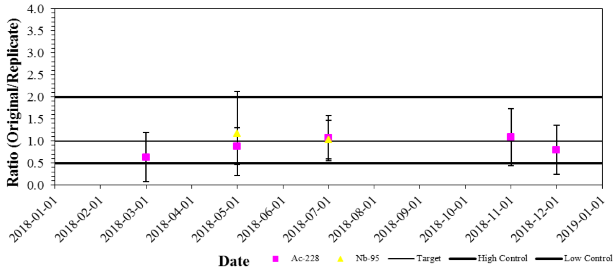
Image 7.12: Performance du niobium-95 et de l'Ac-228 (AQ interne – Double/multiple)
