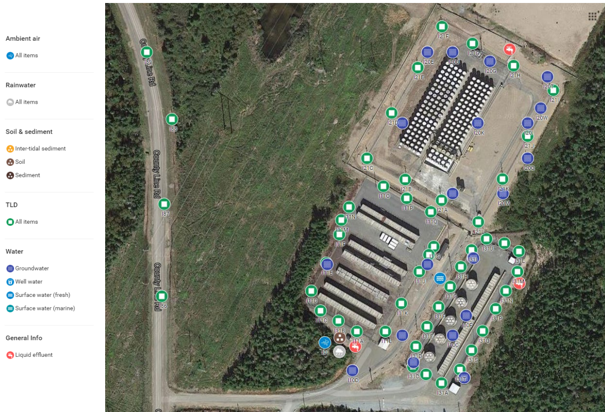
Image 3.06: Surveillance environnementale à l'installation de gestion des déchets radioactifs solides (IGDRS)
