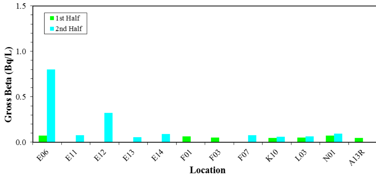
Image 4.11: Radioactivité bêta brute (eau de puits)
