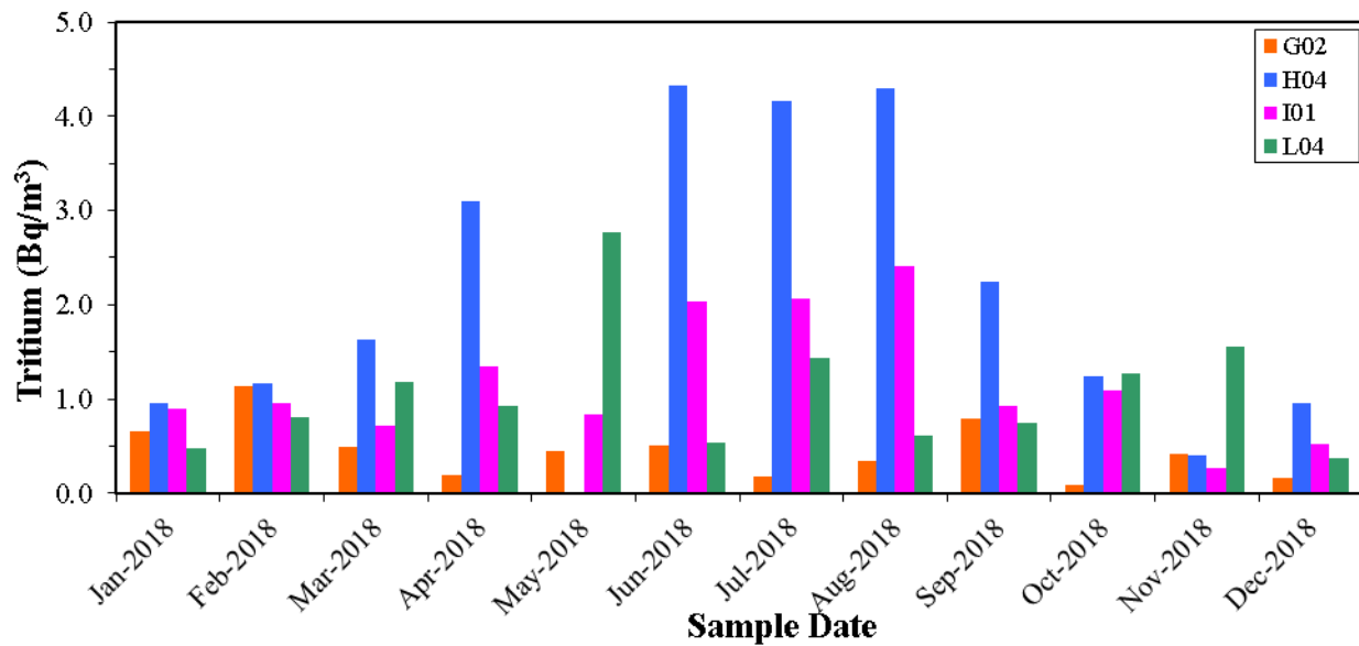
Image 4.04: Tritium (vapeur d'eau) aux postes rapprochés de mesure de la qualité de l'air
