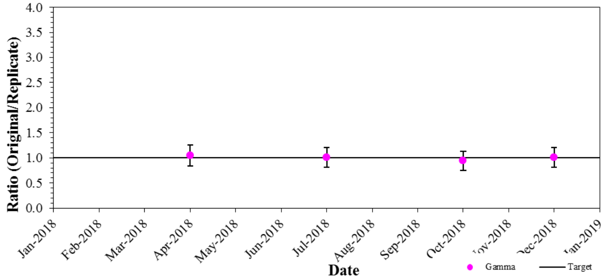
Image 7.09: Performance du rayonnement gamma (AQ interne – Double/multiple)
