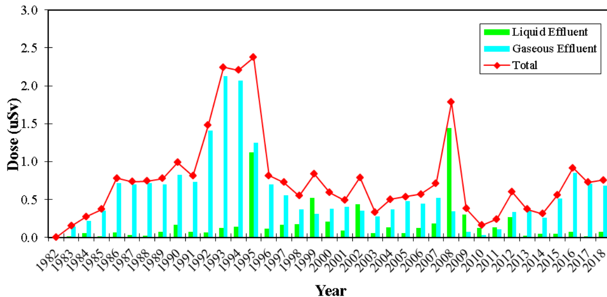
Image 5.1 : Doses mesurées dans l'air et dans les liquides
