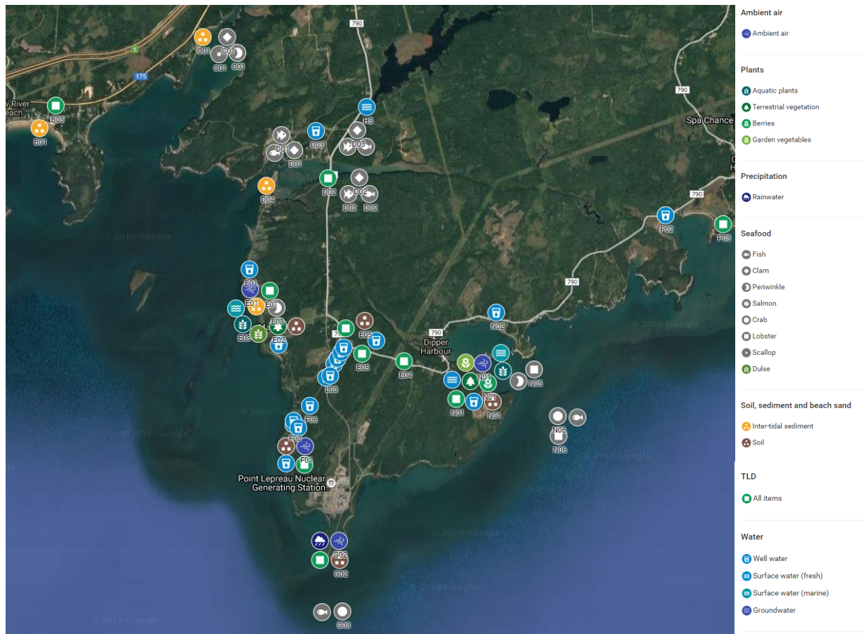
Image 3.05: Surveillance environnementale à la péninsule Lepreau
