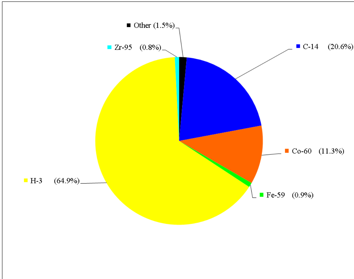
Image 6.02: Contribution des radionucléides à la dose totale (dans les liquides) – 2018
